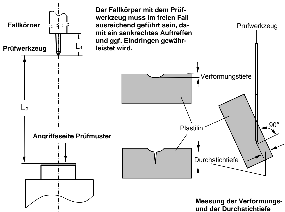
Zeichnung 4: Fallprüfgerät
