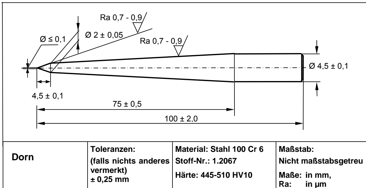
Zeichnung 2: Dorn
