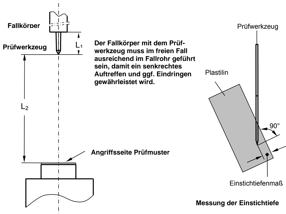
Zeichnung 4: Fallprüfgerät
