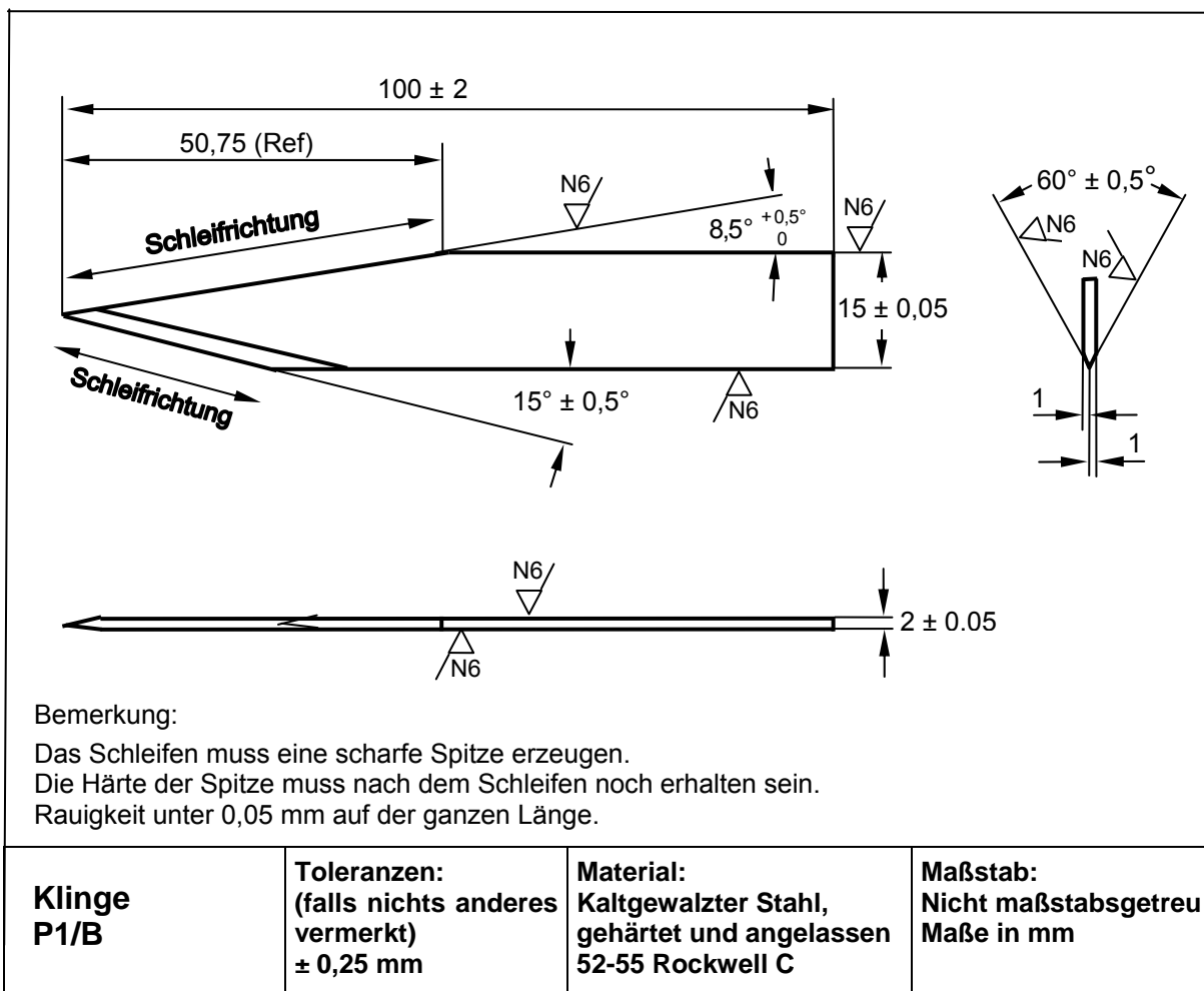
Zeichnung 1: Klinge
